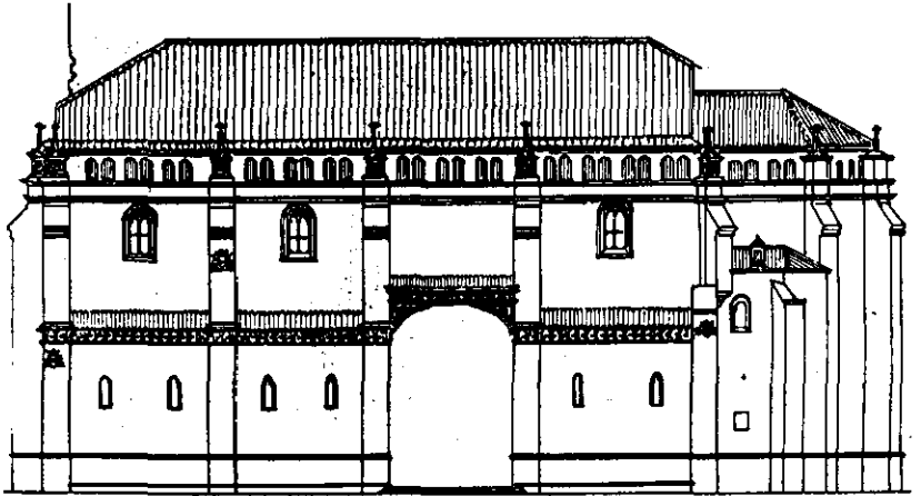
Alzado parcial del templo parroquial de Yepes
