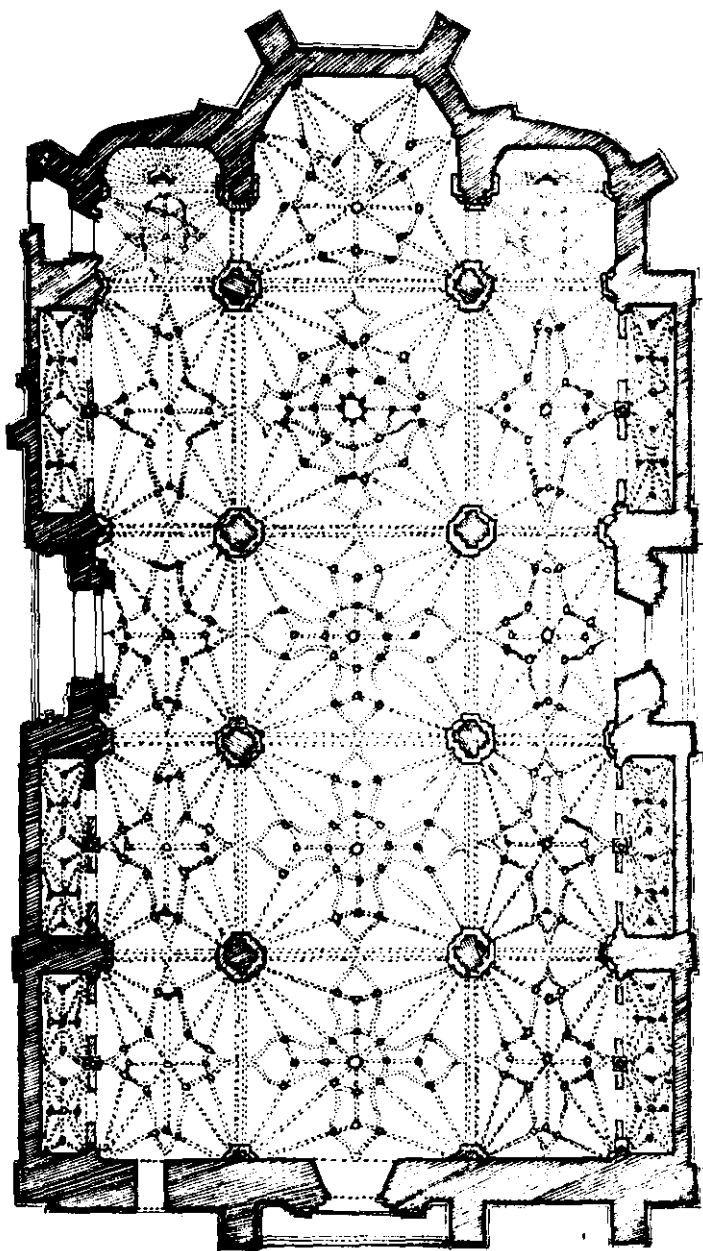
Planta del templo parroquial de Yepes
